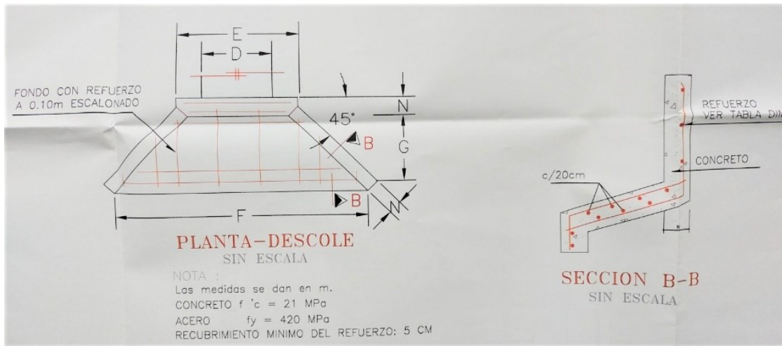
Detalles de las obras del cabezal de descarga. Dimensiones varían según diámetros de tubería de colector. Fuente NF Construarte S.A.S. 2021.
