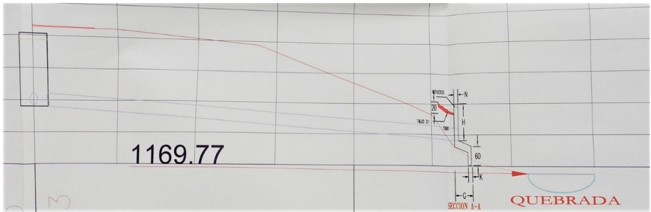
Detalle del perfil de descarga 16 pulgadas respecto a cauce de la quebrada. Fuente NF Construarte S.A.S. 2021.
