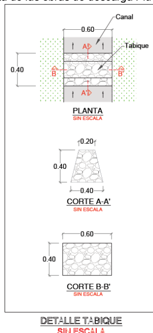
Detalle de las obras de control de velocidad en el canal de descarga. Fuente Tenorio Arzayus. 2021.
