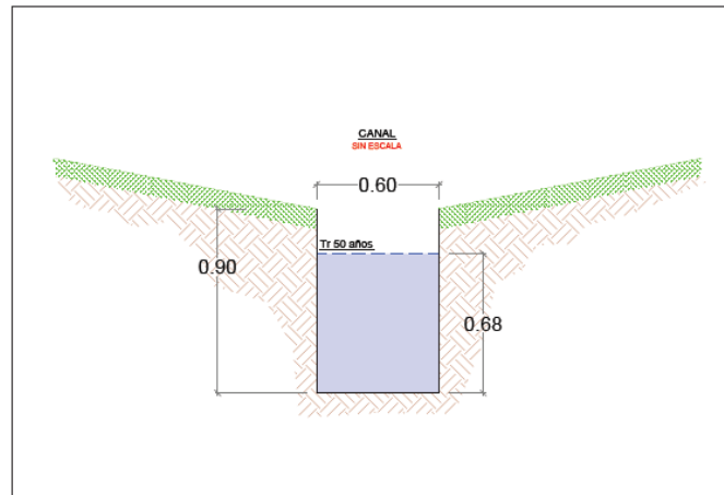
SECCION CANAL PROYECTADO SIN ESCALA
