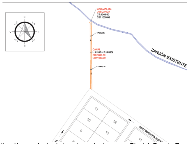
Detalle de la localización en planta de las obras de descarga Pluvial. Fuente Tenorio Arzayus. 2021.
