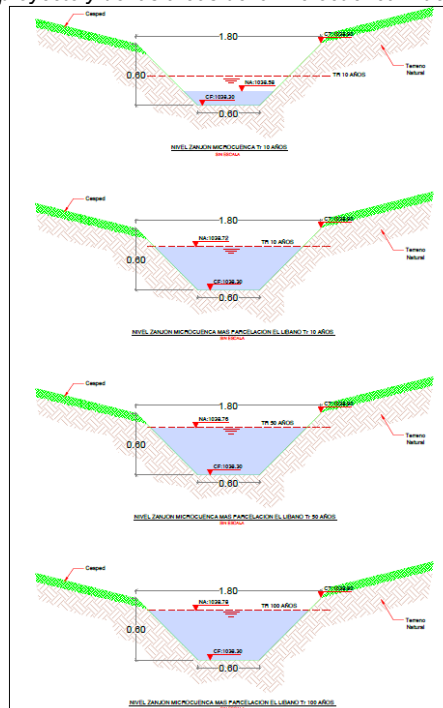
Chequeo de caudales en el zanjón actual. Fuente Tenorio Arzayus. 2021.
