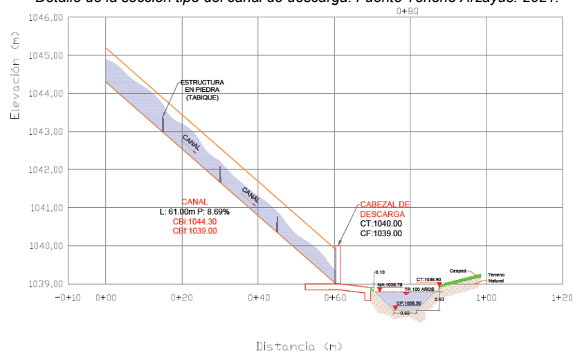
PERFIL CANAL RECTANGULAR PROYECTADO
