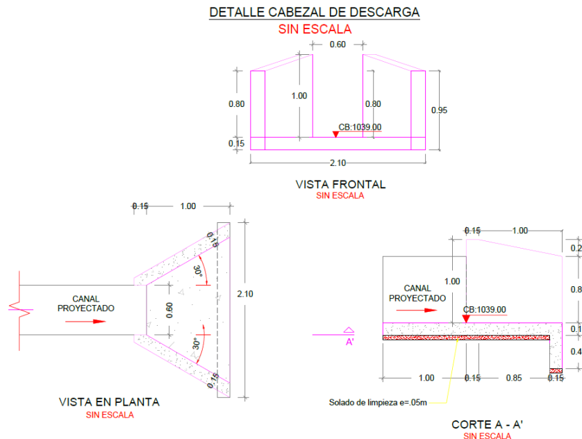
Detalles del cabezal de descarga propuesto. Fuente Tenorio Arzayus. 2021..
